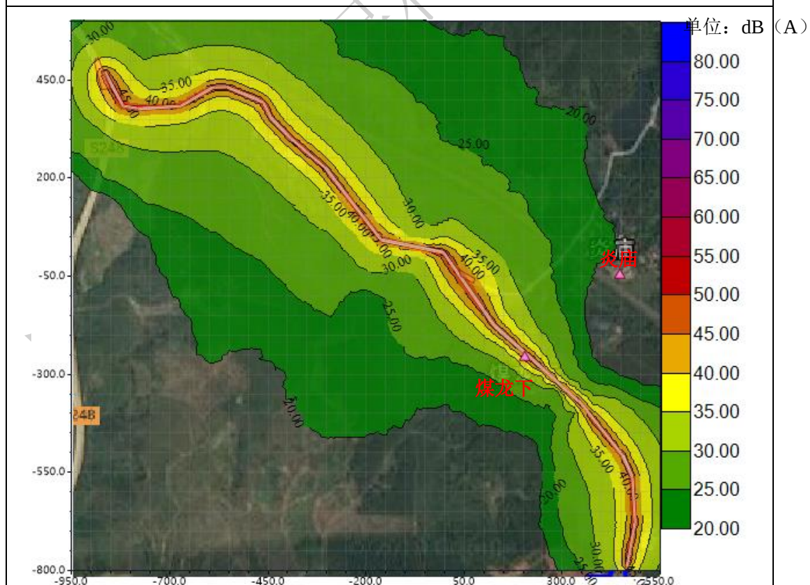
2026 年夜间等声级曲线图 (平均值)
