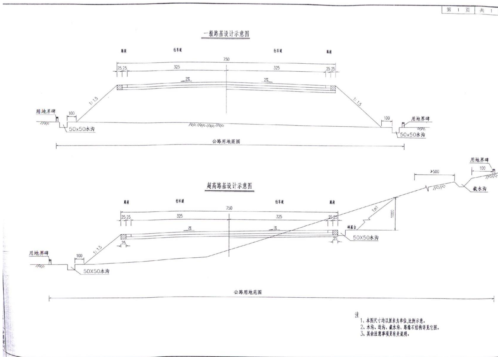
图 3 路基标准断面图
